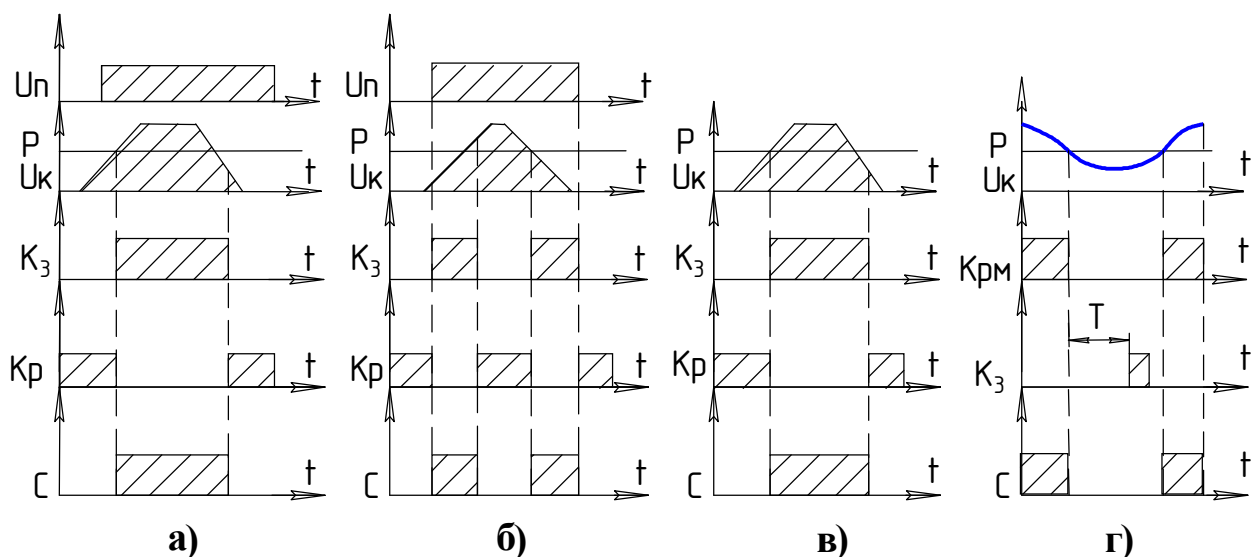
U_n – напряжение оперативного питания; U_k – контролируемое напряжение; P – регулируемый уровень напряжения срабатывания или отпускания; K_з – замыкающий контакт; K_р – размыкающий контакт; K_{рм} – размыкающий контакт мгновенного действия; \zeta – светодиод а) - НЛ4; б) - НЛ5; в) - НЛ6, НЛ7; г) - НЛ11
