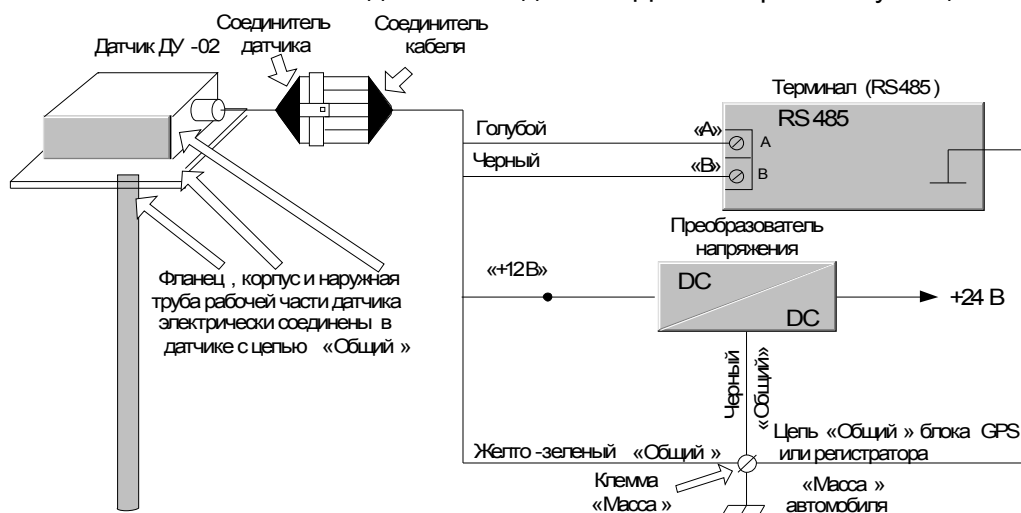
Рис. 2. Схемы подключения датчика ДУ-02 в режимах калибровки, тарировки и штатной работы (при эксплуатации).
