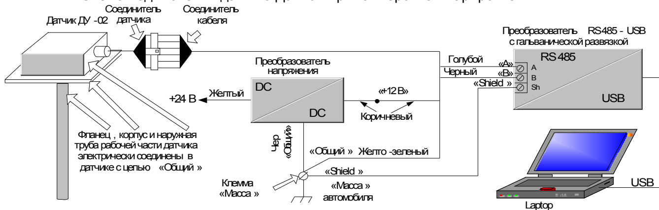
Схема подключения датчика ДУ -02 при эксплуатации
